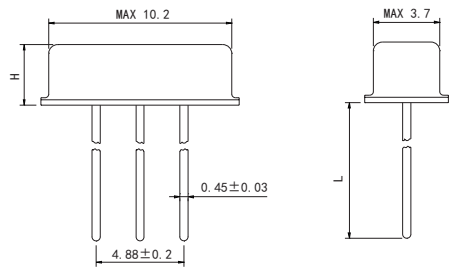
SB: THREE LEADS (三引线) UNIT (单位): mm (毫米)
