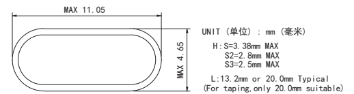
SB: THREE LEADS (三引线) UNIT (单位): mm (毫米)
