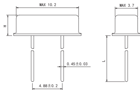
S: TWO LEADS (两引线) UNIT (单位): mm (毫米)
